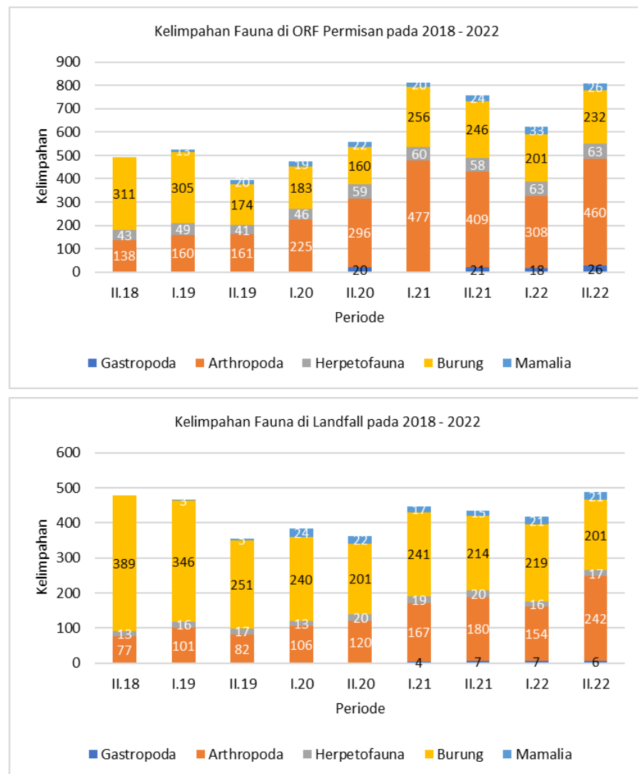
Gambar 3.14 Grafik ilustrasi dinamika kelimpahan fauna di area ORF (gambar atas) dan Landfall (gambar bawah) PT Pertamina Gas OEJA pada tahun 2018 hingga 2022. Periode: I.2018 (semester pertama 2018); II.2018 (semester kedua 2018); I.2019 (semester pertama 2019); II.2019 (semester kedua 2019); I.2020 (semester pertama 2020); II.2020 (semester kedua 2020); I.2021 (semester pertama 2021); II.2021 (semester kedua 2021); II.2022 (semester pertama 2022); II.2022 (semester kedua 2022)
