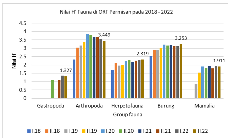
Gambar 3.18 Grafik ilustrasi dinamika nilai indeks diversitas Shannon-Wiener ( H' ) komunitas fauna di area ORF PT Pertamina Gas OEJA pada tahun 2018 hingga 2022. Periode: I.2018 (semester pertama 2018); II.2018 (semester kedua 2018); I.2019 (semester pertama 2019); II.2019 (semester kedua 2019); I.2020 (semester pertama 2020); II.2020 (semester kedua 2020); I.2021 (semester pertama 2021); II.2021 (semester kedua 2021); I.2022 (semester pertama 2022); II.2022 (semester kedua 2022)
