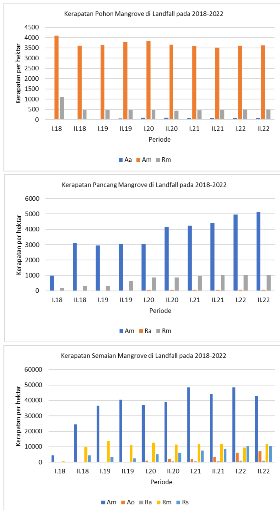
Gambar 3.7 Grafik ilustrasi dinamika kerapatan tegakan pohon (gambar atas), pancang (gambar tengah) dan semaian (gambar bawah) mangrove di area Landfall PT Pertamina Gas OEJA pada tahun 2018 hingga 2022. Spesies: Aa. Avicennia alba ; Am. A. marina ; Ao. A. officinalis ; Ra. Rhizophora apiculata ; Rm. R. mucronata ; Rs. R. stylosa
