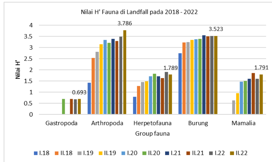
Gambar 3.19 Grafik ilustrasi dinamika nilai indeks diversitas Shannon-Wiener ( H' ) komunitas fauna di area Landfall PT Pertamina Gas OEJA pada tahun 2018 hingga 2022. Periode: I.2018 (semester pertama 2018); II.2018 (semester kedua 2018); I.2019 (semester pertama 2019); II.2019 (semester kedua 2019); I.2020 (semester pertama 2020); II.2020 (semester kedua 2020); I.2021 (semester pertama 2021); II.2021 (semester kedua 2021); I.2022 (semester pertama 2022); II.2022 (semester kedua 2022)
