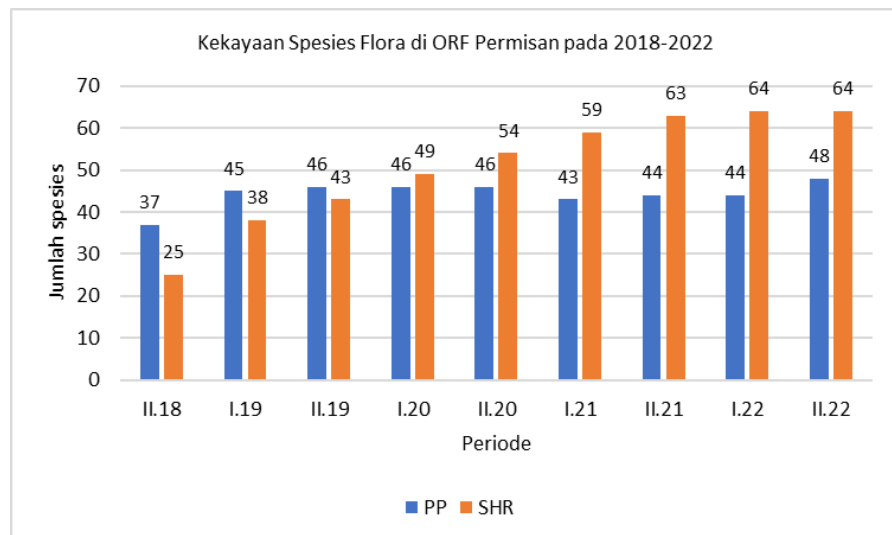
Gambar 3.3 Grafik ilustrasi dinamika kekayaan spesies flora di area ORF PT Pertamina Gas OEJA pada tahun 2018 hingga 2022. Keterangan: PP . kategori tegakan pohon dan palem; SHR . kategori tegakan semak, herba dan rumput
