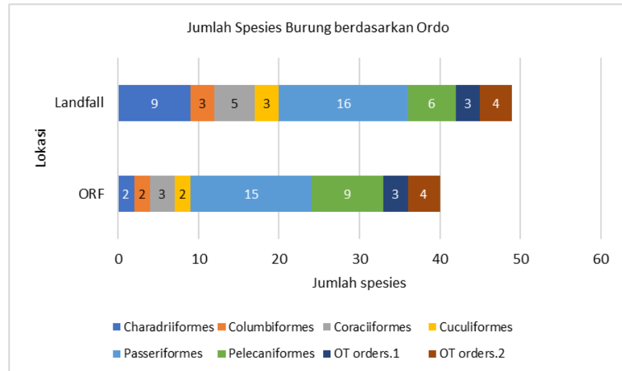
Gambar 3.16 Proporsi jumlah spesies burung berdasarkan ordo atau bangsa di area ORF dan Landfall PT Pertamina Gas OEJA di Jabon, Sidoarjo pada semester kedua 2022. OT orders: ordo yang diwakili oleh 1 atau 2 spesies
